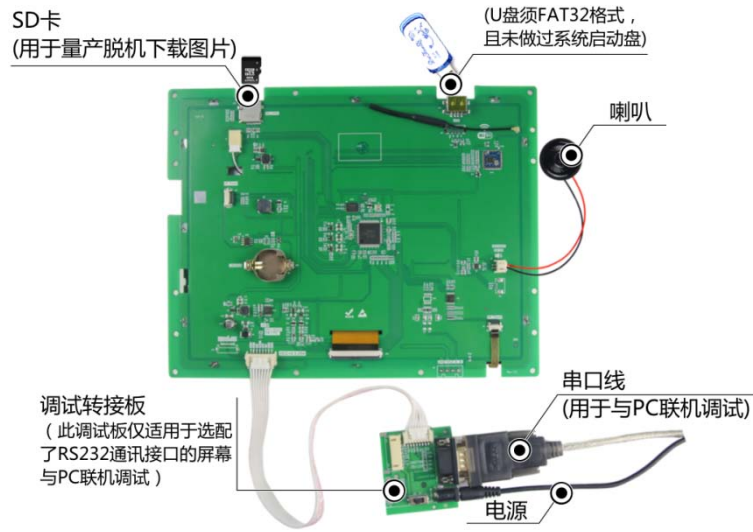
图 1-5 调试工具
