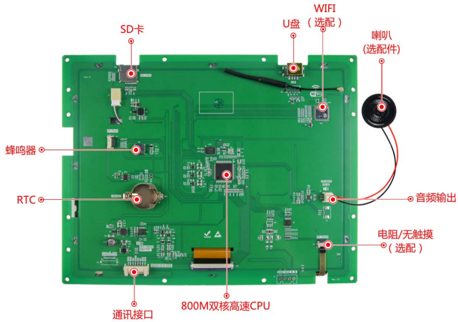
图 1-3 硬件配置图
