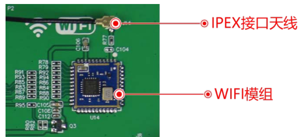
图 1-4 WIFI 配置图
